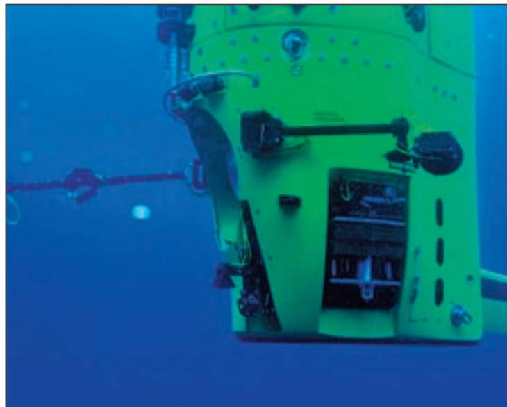
El submarino Deepsea Challenger y su brazo robótico
