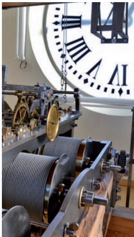
Mecanismo del reloj de Sol, que cumple 150 años
