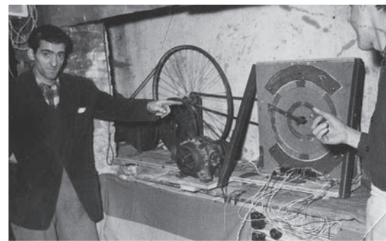
Mecanismo del belén del bar Bilbao, año 1955.
